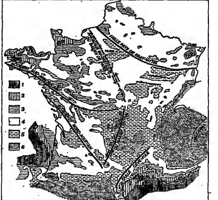
1. Anomalie positive supérieure à +20 milligals. 2. Anomalie positive comprise entre +5 et +20 milligals. 3. Anomalie comprise entre -5 et +5 milligals. 4. Anomalie négative comprise entre -25 et -5 milligals. 5. Anomalie négative comprise entre -45 et -25 milligals. 6. Anomalie négative supérieure à -45 milligals. Les courbes indiquent le sens du coulisage. Toutes ces anomalies sont calculées par rapport à la valeur théorique de la pesanteur. Cette valeur théorique a été calculée pour une Terre homogène qui aurait la forme d'un globe parfait. Le milligal est la millièmes partie du gal, unité d'accélération adimensionnelle sur l'accélération de pesanteur (981 cm/sec.² en moyenne). La carte ci-dessus est une version simplifiée du document publié par le B.R.G.M. Sur la carte au 1:1 000 000, les courbes d'anomalies sont tracées pour chaque milligal, ce qui rend les grands accidents beaucoup plus visibles que sur notre carte.
